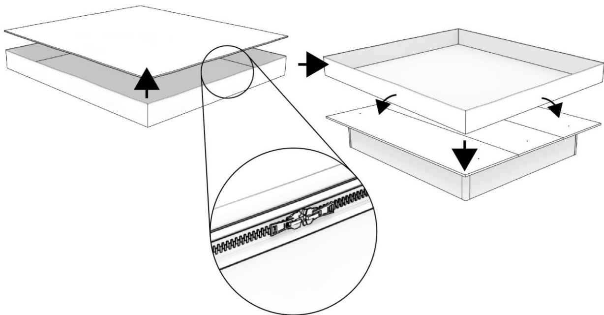
Figuur 9: Loskoppelen van bovenkant en onderkant tijk, omvouden van de randen van de onderste tijk over de bodemplaten heen. Ritssluiting komt aan het voeteind.
