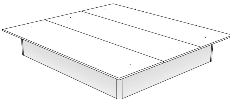
Figuur 6: Plaatsen van de 2 e en 3 e bodemplaat op het bedbodem.
