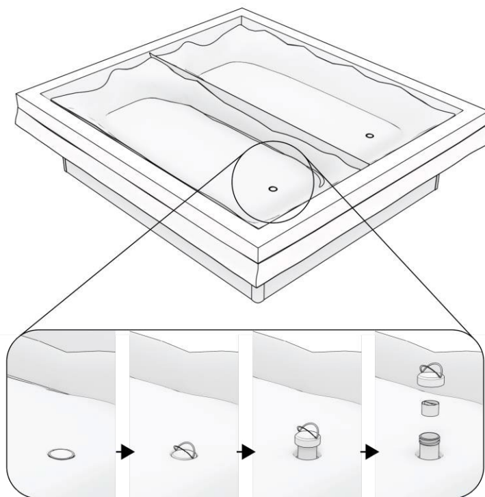
Figuur 15: Positionering van de watermatrassen en openen van de vuldoppen.
