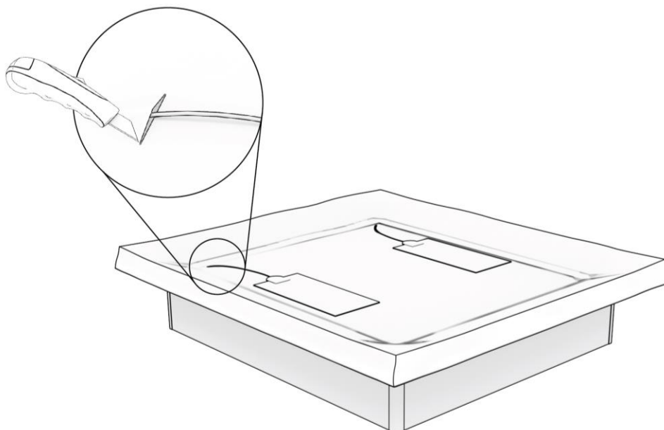
Figuur 9: Positionering van de verwarmingselementen en doorvoersleuven snijden in de bodem tijk.
