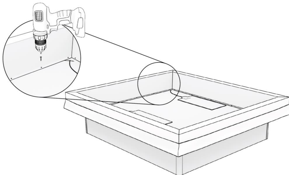
Figuur 12: Vastschroeven van de schuimrandlatten aan de bodemplaten.
