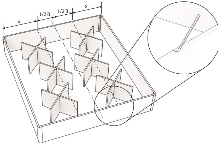
Figuur 4: Teken van hartlijn op kop- en voeteind van het bedbodem.
