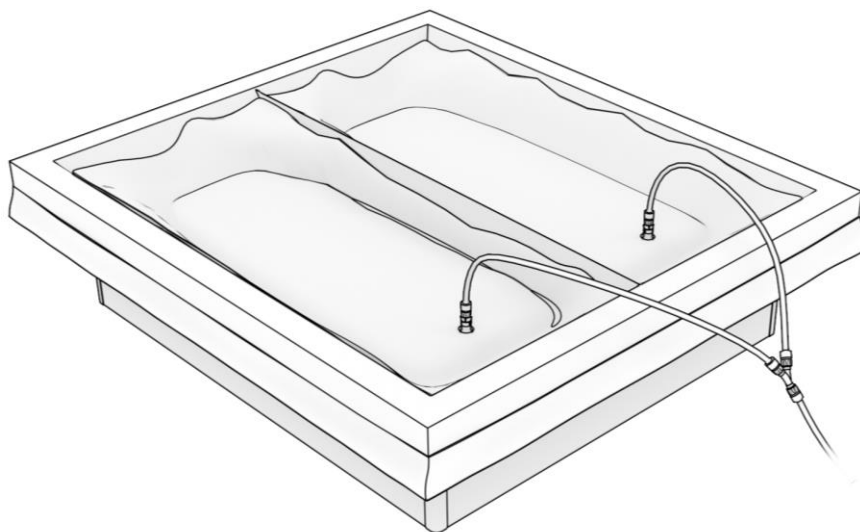
Figuur 16: Koppelen van de vulslang aan het watermatras om het matras te vullen met water.
