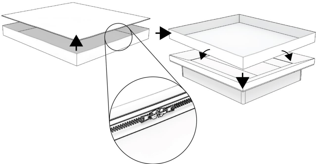
Figuur 8: Loskoppelen van bovenkant en onderkant tijk, omvouwden van de randen van de onderste tijk over de schuimranden heen. Ritssluiting komt aan het voeteind.
