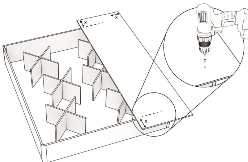
Figuur 5: Plaatsen en vastschroeven van de 1 e bodemplaat op het bedbodem.
