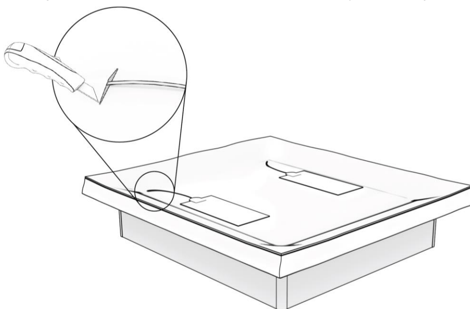
Figuur 10: Plaatsen van de isolatiemat, positionering van de verwarmingselementen en doorvoersleuven snijden in de isolatiemat.
