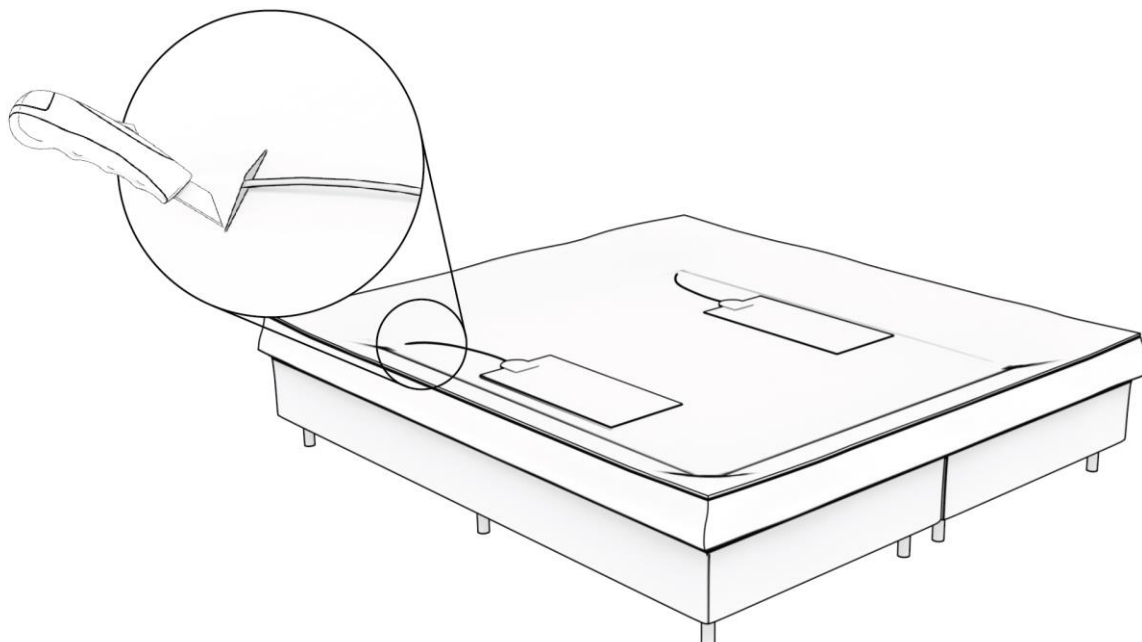
Figuur 7: Plaatsen van de isolatiemat, positionering van de verwarmingselementen en doorvoersleuven snijden in de isolatiemat.
