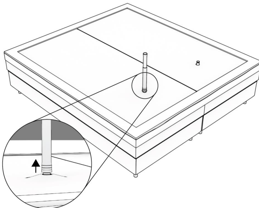
Figuur 16: Het laatste lucht uit het watermatras pompen met de ontluuchtingspomp.
