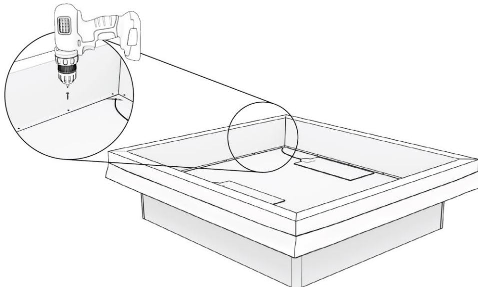
Abbildung 12: Verschrauben der Schaumrandlatten mit den Bodenplatten.
