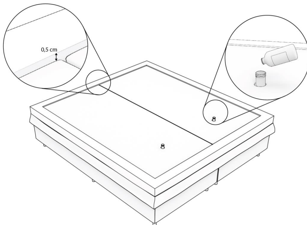
Abbildung 14: Wassermatratze bis 0,5 cm unterhalb des Schaumrandes gefüllt und in beiden Matratzen Konditionierer hinzugefügt.
