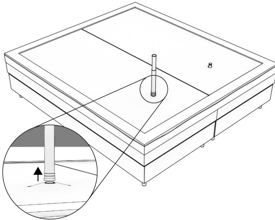
Abbildung 16: Die letzte Luft mit der Entlüftungspumpe aus der Matratze pumpen.
