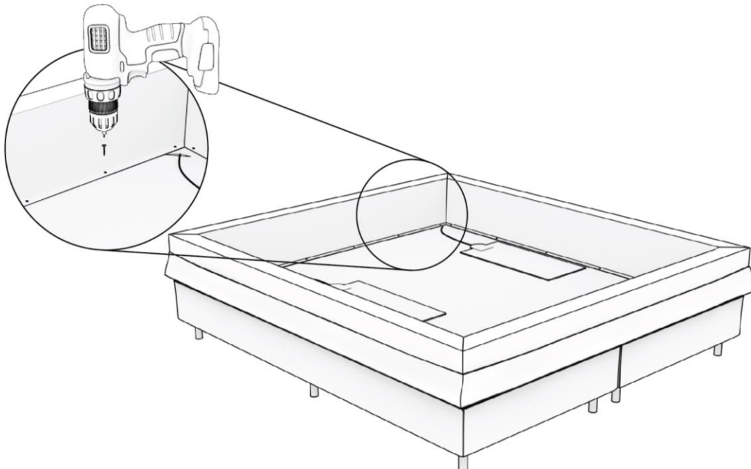
Abbildung 9: Verschrauben der Schaumrandlatten mit den Bodenplatten.
